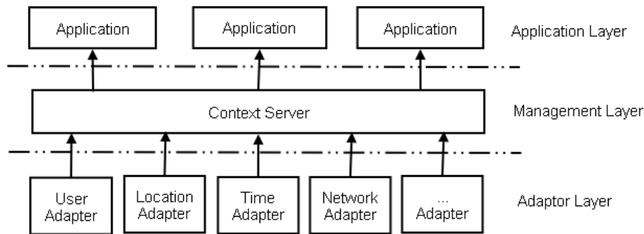
Figura 3.7: Arquitetura do Hydrogen (HOFER et al., 2002)
