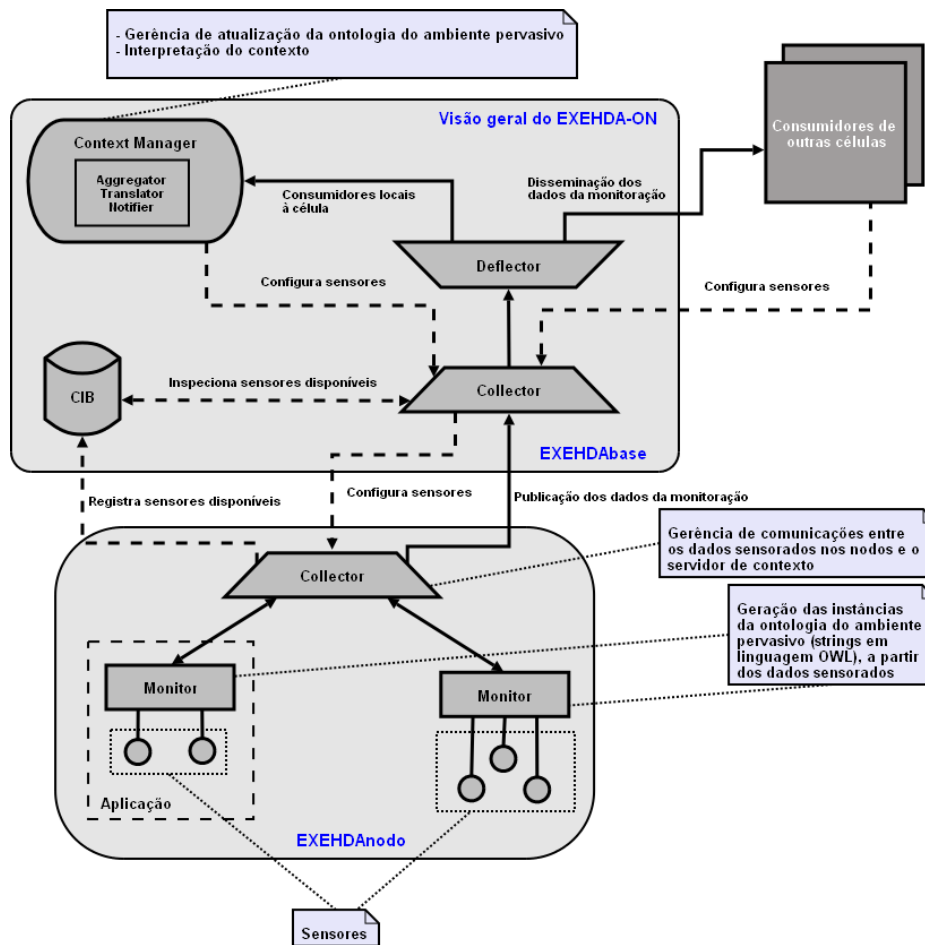
Figura 5.5: Integração das funcionalidades do EXEHDA-ON
