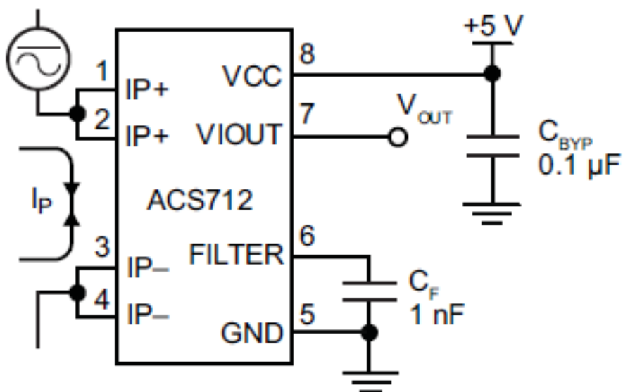
ACS712
